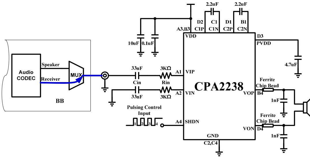
图 5 CPA2238Receiver 模式典型应用图
