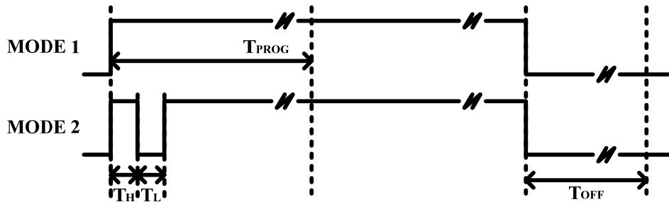
图 12 一线脉冲控制方法示意图
