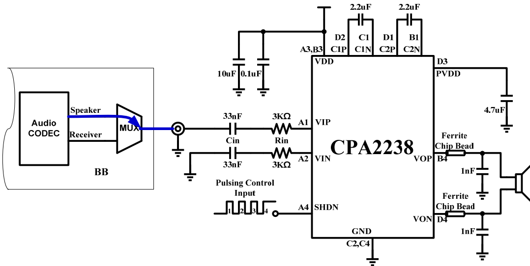
图 4 CPA2238Speaker 模式典型应用图
