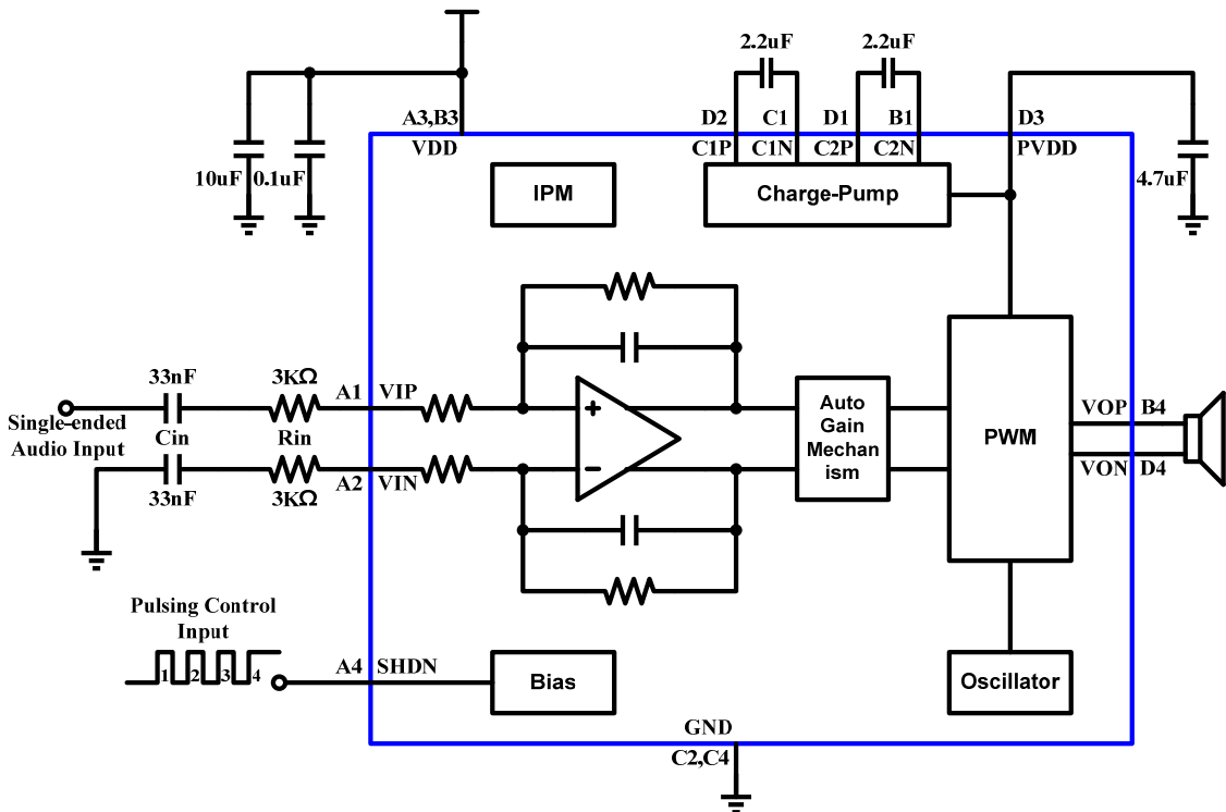
图 17 单端输入的典型应用示意图
