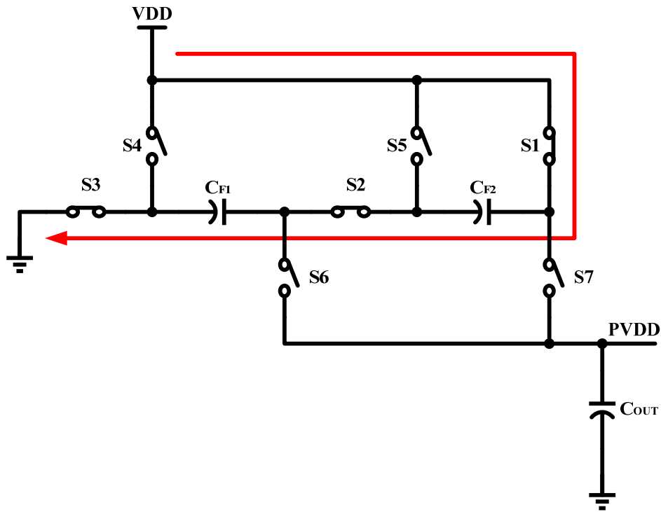
图 8 充电相电流通路示意图
