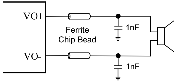
图 14 典型磁珠、电容滤波电路示意图
