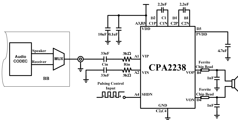
图 1 CPA2238 差分输入典型应用图
