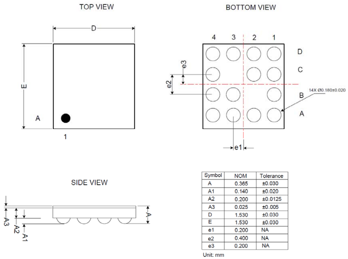
图 18 WLCSP14 1.53mmx1.53mm Package
