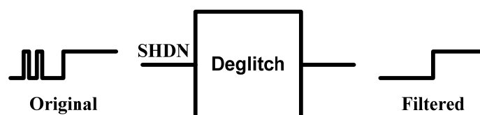
图 10 复合毛刺消除技术示意图
