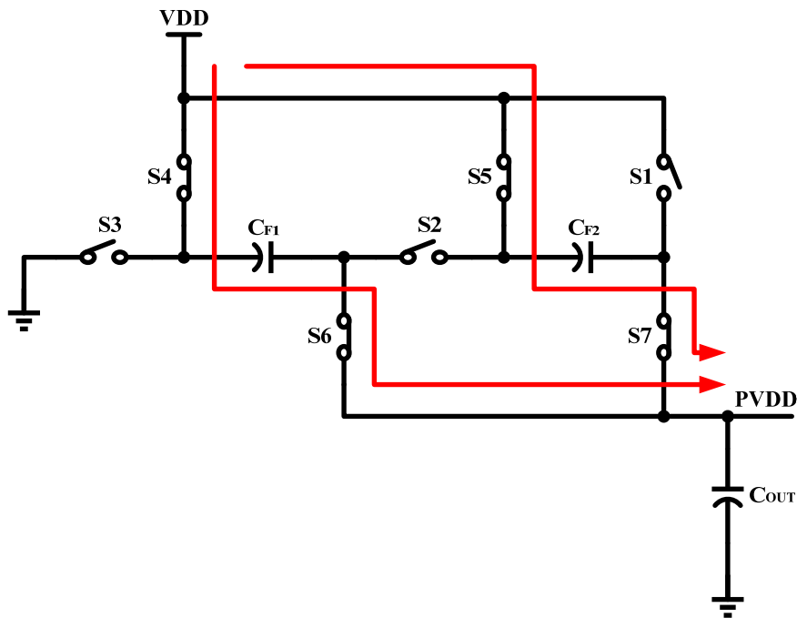
图 9 输出相电流通路示意图
