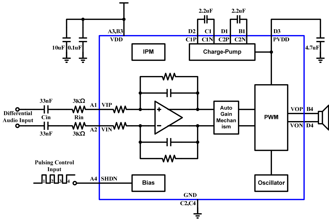
图 3 CPA2238 差分输入典型应用图
