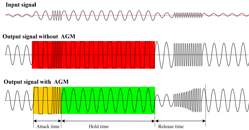
图 6 自动增益管理功能原理图
