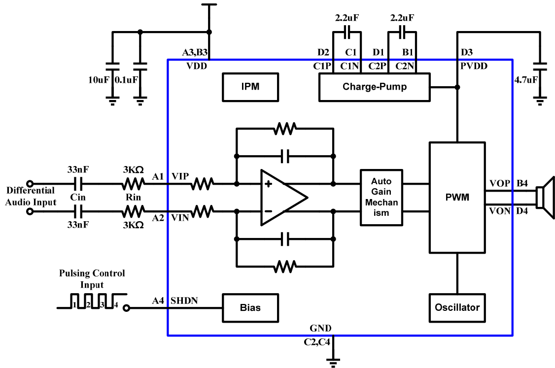
图 16 差分输入的典型应用示意图
