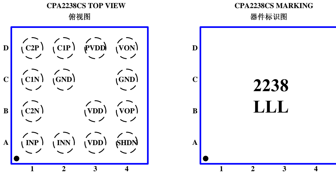
图2 CPA2238CS 引脚分布俯视图及器件标识图
