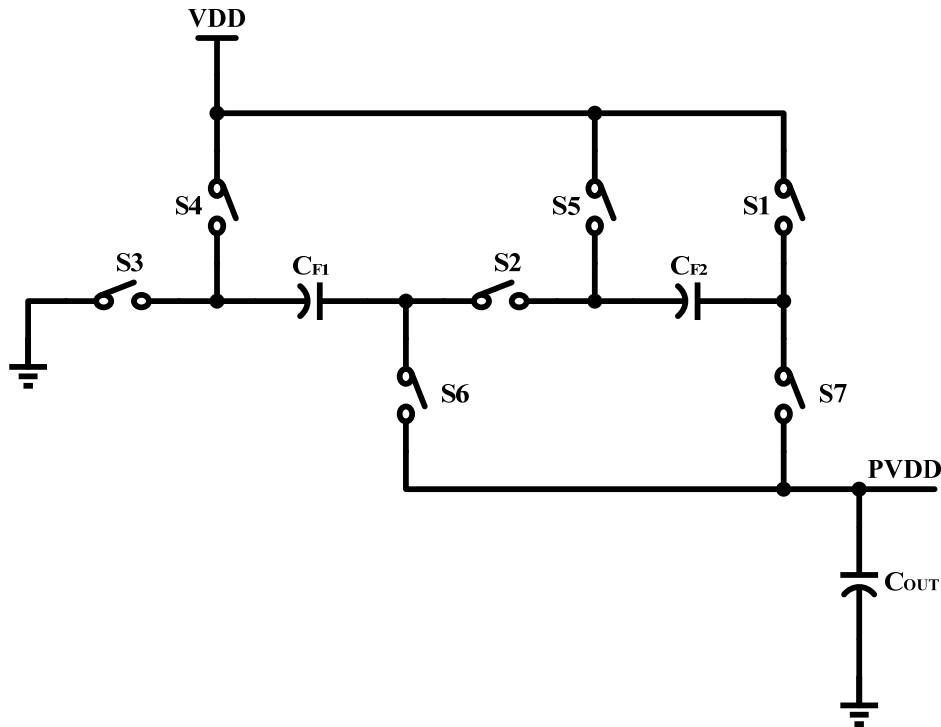
图 7 1.5 倍电荷泵原理图
