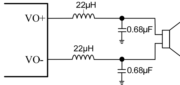
图 15 典型 LC 滤波电路示意图
