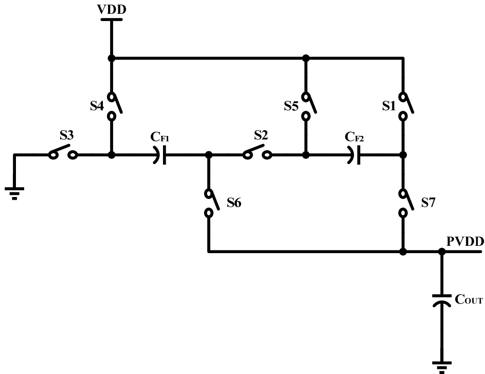
图 7 1.5 倍电荷泵原理图
