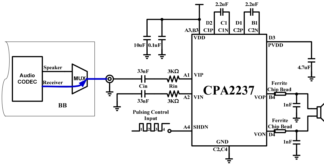
图 5 CPA2237Receiver 模式典型应用图
