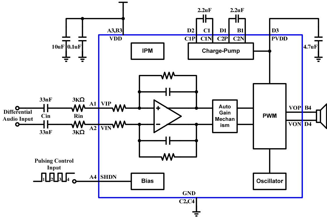
图 3 CPA2237 差分输入典型应用图
