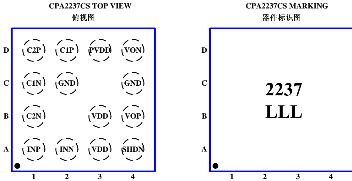
图 2 CPA2237 引脚分布俯视图及器件标识图
