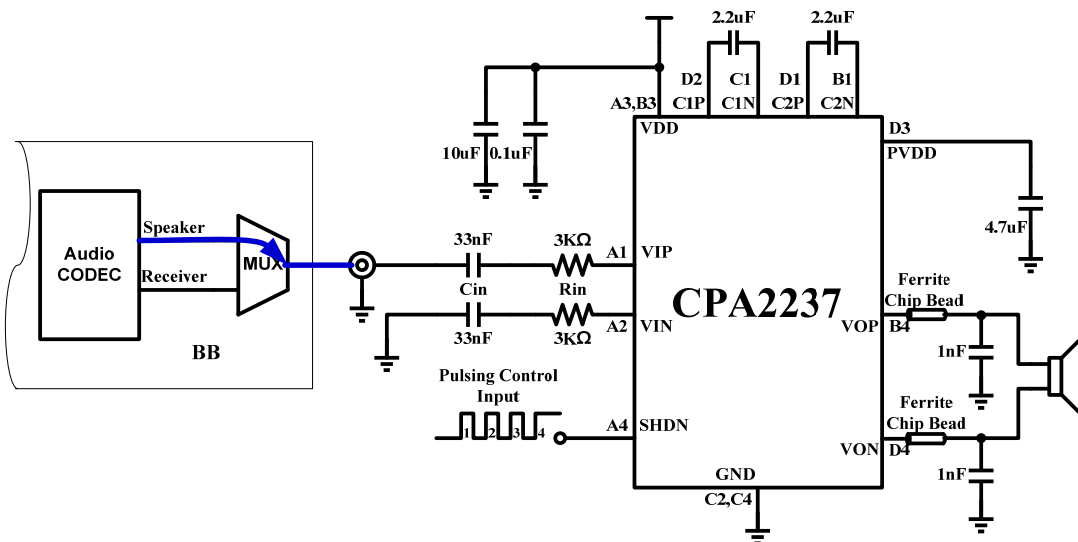
图 4 CPA2237 Speaker 模式典型应用图
