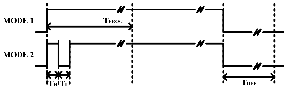
图 12 一线脉冲控制方法示意图
