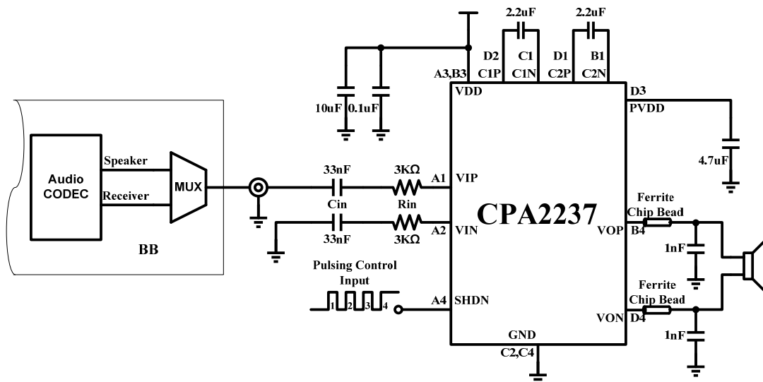
图 1 CPA2237 差分输入典型应用图
