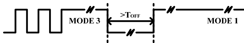
图 13 模式切换时序控制示意图
